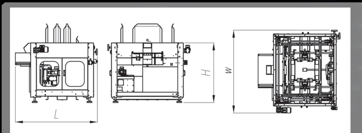
Machine : Dimensions // en millimètres
